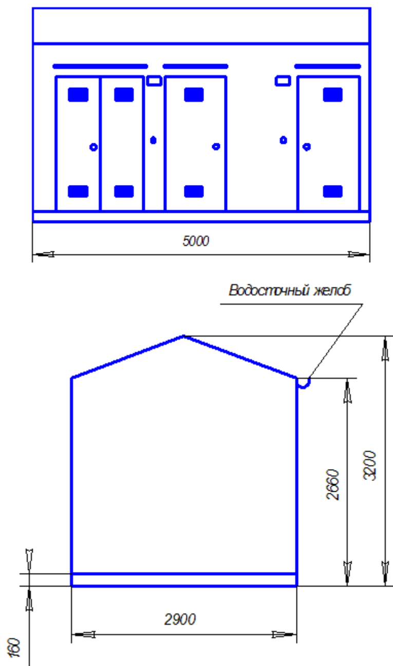
Рис 1. Габариты БМС-ЭРА-ЮНЭП. Исполнение воздух, кабель
