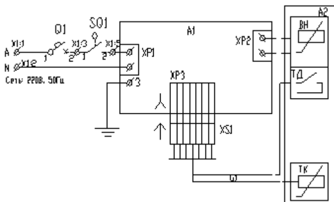
Схема электрическая шкафов ВШОВ
