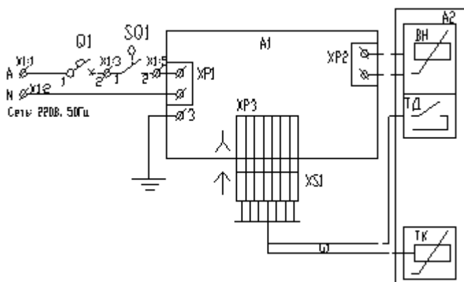
Схема электрическая шкафов ВШОЭ
